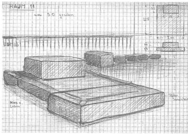
Abb. 8 Augst, Insula 24 (Grabung 1939.51). Drei-dimensionale Ansicht der Befundsituation im Bereich der als Schlachtbank interpretierten Sandstein-Konstruktion in Raum A. Im Hintergrund ist die an eine Sandstein-spolie anschliessende «späte» Steinsetzung zu erkennen, auf der höchstwahrscheinlich der Schwellbalken einer Fachwerkwand ruhte. Zur Raumbezeichnung vgl. Anm. 28.
