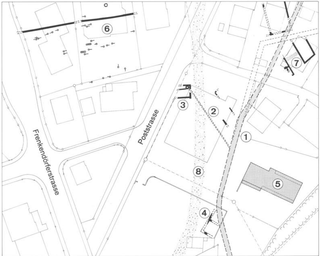
Abb. 19 Augst, Region 10,A (Grabung 1994.58). Archäologischer Situationsplan im Bereich des spätmittelalterlichen Mühlekanales. M. 1:1000.
