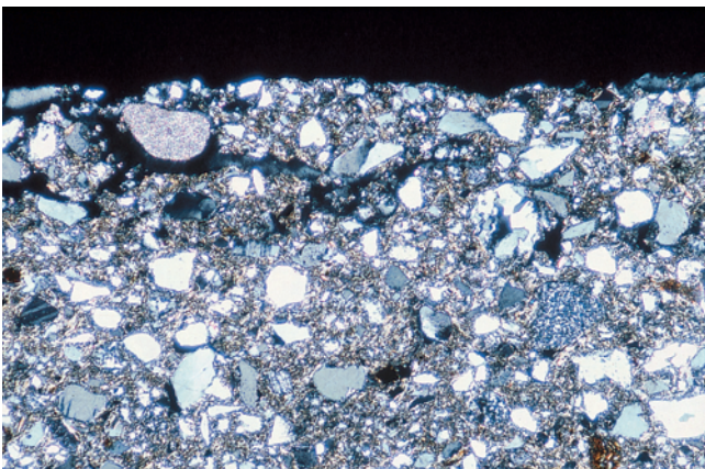
Abb. 4 Mikrofoto der Probe T15, Oberfläche der Schicht a. Zu-stand nach Kompaktion während 15 Minuten, trockenes Substrat. Der kompaktierte Bereich zeichnet sich durch eine sehr geringe Porosität sowie oberflächlich verlaufende, horizontale Risse ab. Weitere Merkmale sind eingeregelter Sandkörner und ein granu-läres Gefüge unter der Grenzfläche. Die gelbe Tonsubstanz ist komplett aufgearbeitet und befindet sich ausschliesslich in der Matrix. Bildbreite 2,2 mm, XPL.
