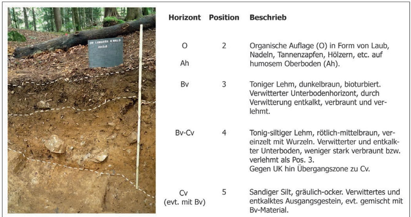
Abb. 11. Lungern OW, Balmiwald, Römerplätzli (= Abb. 1,5). Sondierschnitt S1, Profil P1. Feldaufnahme S. Brunner und A. Wicki; Foto S. Brunner; Ausarbeitung und geoarchäologische Interpretation T. Lander.
