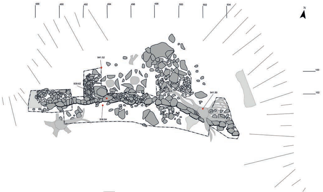
Abb. 6. Lungern OW, Balmiwald, Letzi (= Abb. 1,2). Aufsicht der mittelalterlichen oder (früh)neuzeitlichen Letzimauer. Feldaufnahme J. Bucher; Umsetzung P. Nagy/D. Schuhmann.
