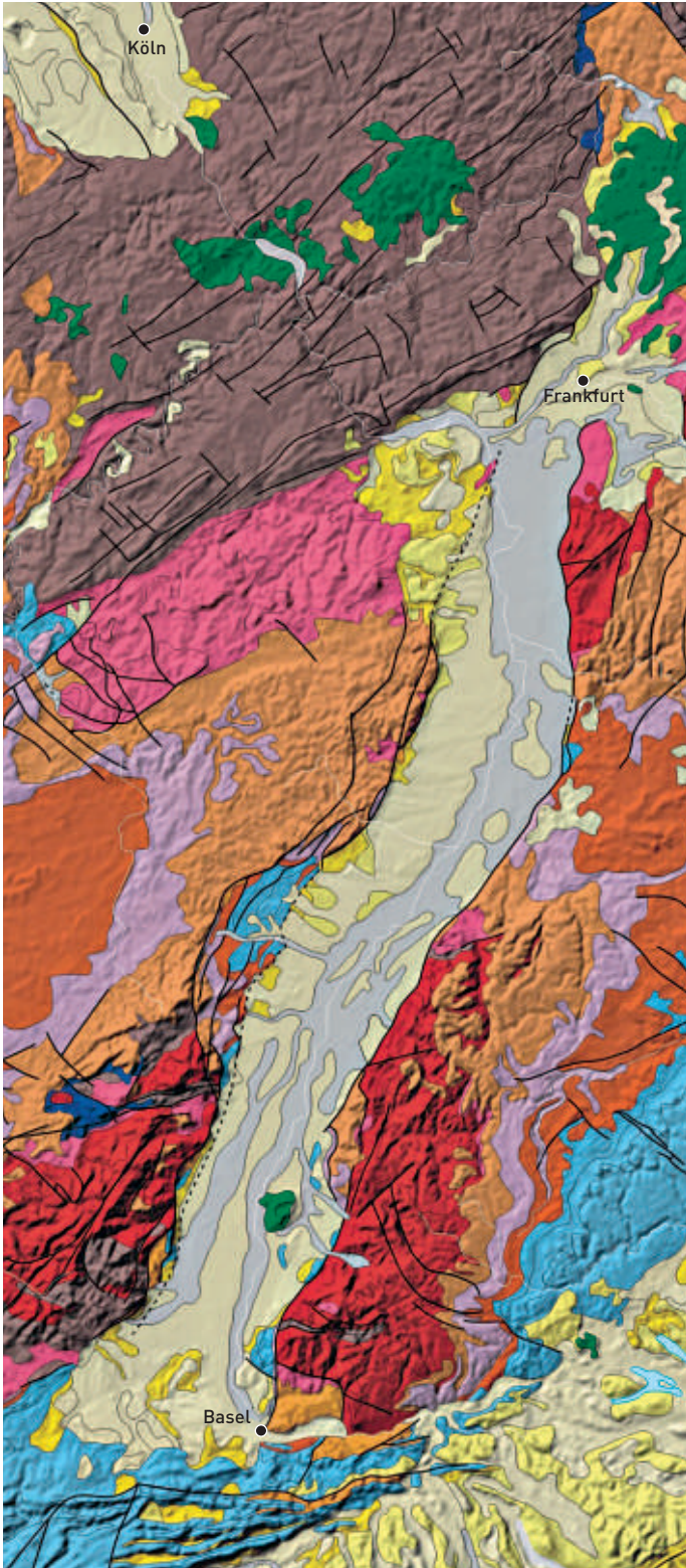
ABB 3.1 Geologische Situation heute. Die Lücke zwischen den auseinandergedrifteten Gebirgszügen des Grundgebirges (dunkelrot, Schwarzwald und Vogesen) wird durch tertiäre Schwemmsedimente verfüllt (gelb). Während dem Oligozän gab es mehrere Vulkane, die heute nicht mehr aktiv sind (z. B. der Kaiserstuhl, grün). Südlich von Basel schliesst der Tafel- und Faltenjura an (hellblau).
